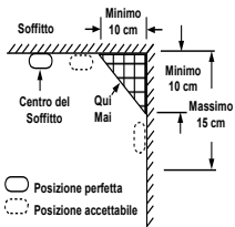
Figura 3: Posizioni perfetta e accettabile di installazione dei rivelatori di fumo e di calore.
