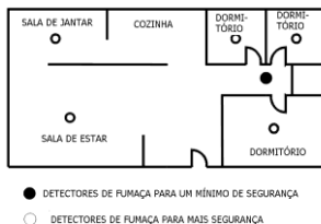
Figura 1: Locais de instalação para detectores de fumo e calor em apartamentos ou casas para uma família com apenas uma área de dormitório.
