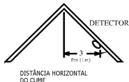
Figura 4: Local de instalação recomendado para detectores de fumo e calor em ambientes com tetos inclinados ou telhados de duas águas (inclinação > 20 graus).
