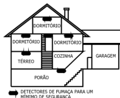
Figura 2: Locais de instalação para detectores de fumo e calor em apartamentos ou casas com mais de um andar.
