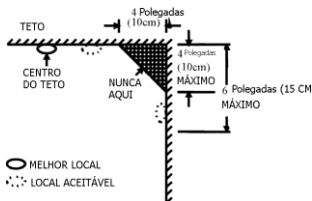
Figura 3: Recomendações para os melhores e mais aceitáveis locais para instalar os detectores de fumo e calor.
