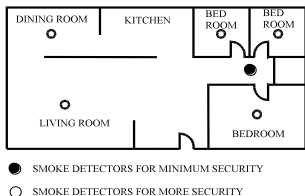
Figuur 1: Installatie van rook & hitte detectoren in een appartement of woning met 1 enkele slaapkamer
