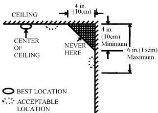
Figuur 3: Aanbevelingen om de rook & hitte detectoren op de best mogelijke locatie te installeren.
