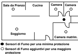
Figura 1: Posizionamento dei rivelatori di fumo e di calore all'interno di una abitazione con una sola zona notte.
