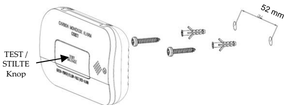
Figuur 2 – Installeren
