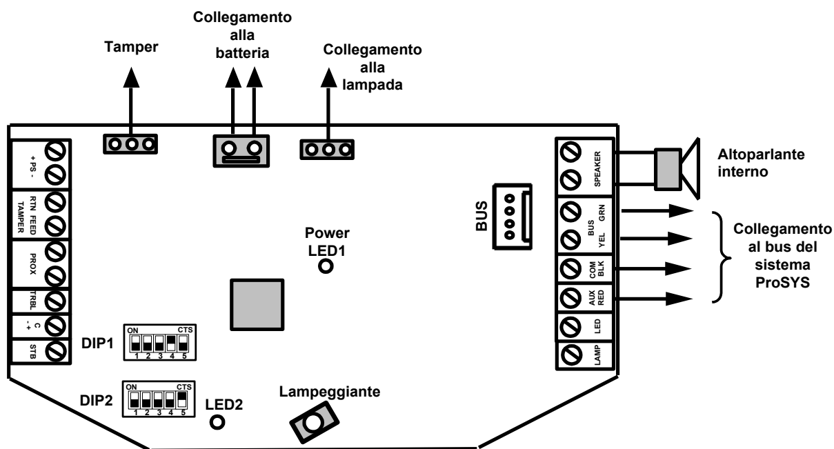
Figura 2 – Configurazione BUS
