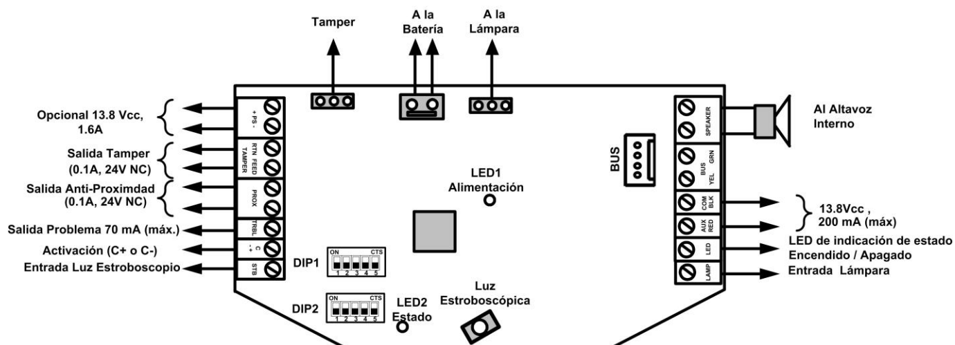
Figura 1 – Cableado en modo “Stand-Alone”
